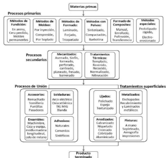
Figura 5. Árbol de clasificación de procesos traducción del original (Ashby, Shercliff, & Cebon, 2014)
